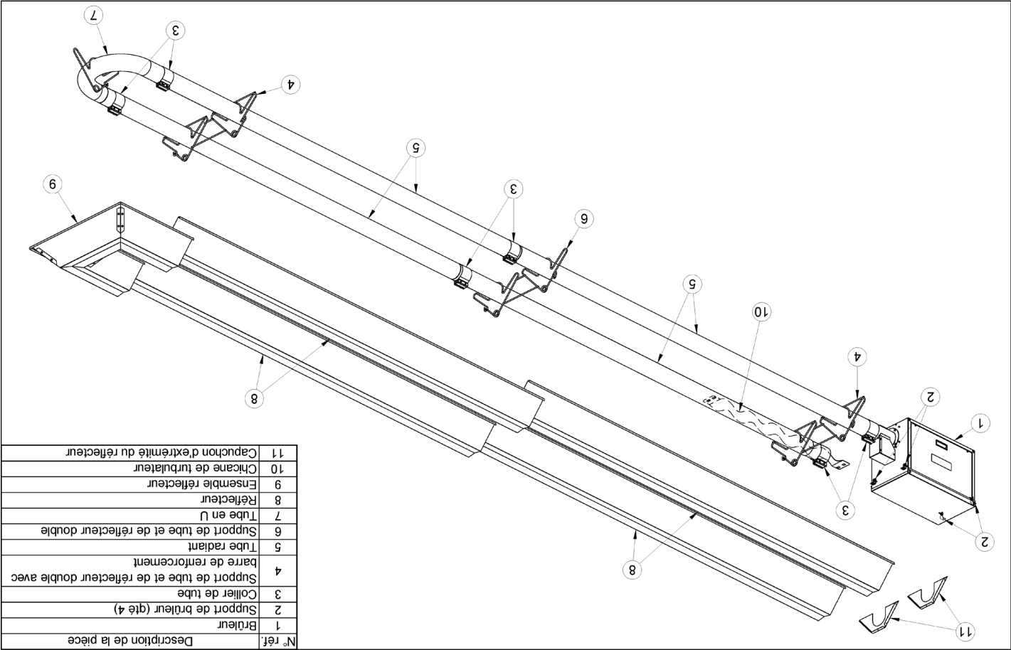
Figure 7.1 - Composants du système de tube en U
