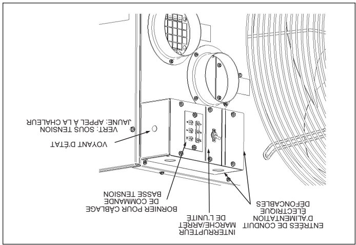
Figure 14.1 - Boîte pratique avec interrupteur à bascule pour entrepreneur
